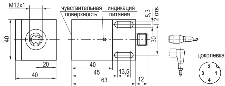
Габаритный чертеж
